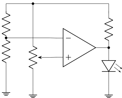
Montage comparateur de base
