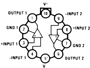
Repérage des broches (TO-100)
